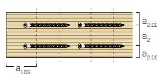
rzut poziomy
