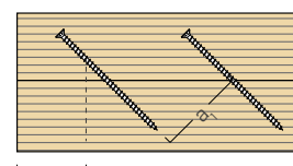
rzut pionowy
