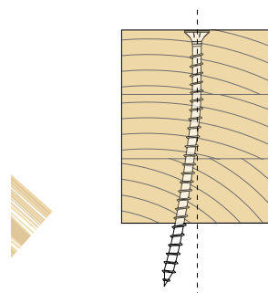
behelyezés vezetőfurat nélkül
