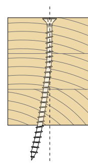
namestitev brez pilotne izvrtine
