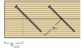
vooraanzicht
