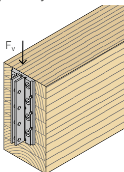
pomocný nosník
