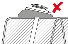
错误拧紧 离轴
