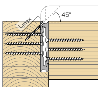
opcionális csavar \varnothing 5 mm - L_{max} = 50 mm
