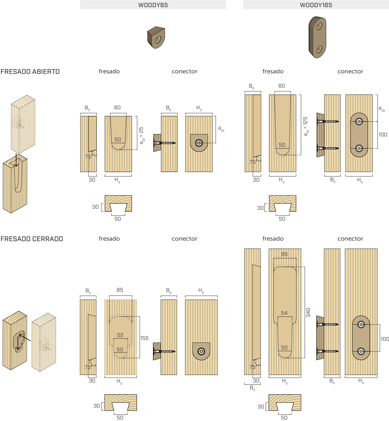
DISTANCIAS Y DIMENSIONES MÍNIMAS
