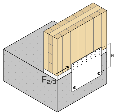
fixação parcial
