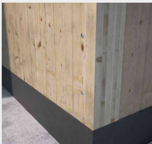
^ ^ Bevestiging SIP-panelen met TBS-schroeven diameter 8 mm. Bevestiging wanden van CLT met schroeven TBS.
