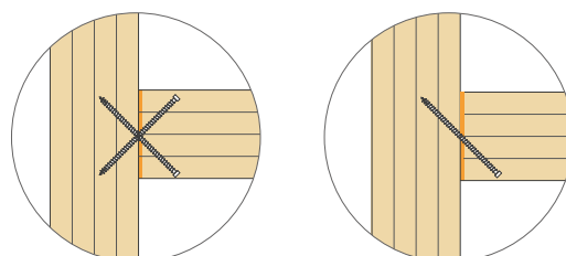
04 Verbindung Treppenaufsatz/durchgehende Wand
