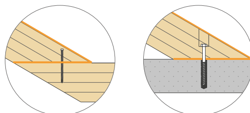
03 Verbindung Antritt Treppe-Treppenaufsatz
