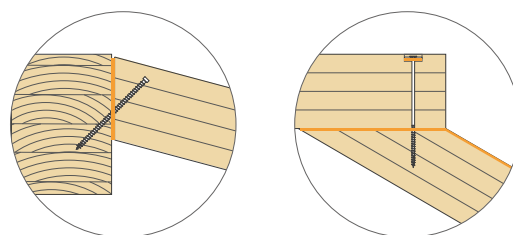
01 Verbindung Austritt Treppe-Treppenaufsatz
